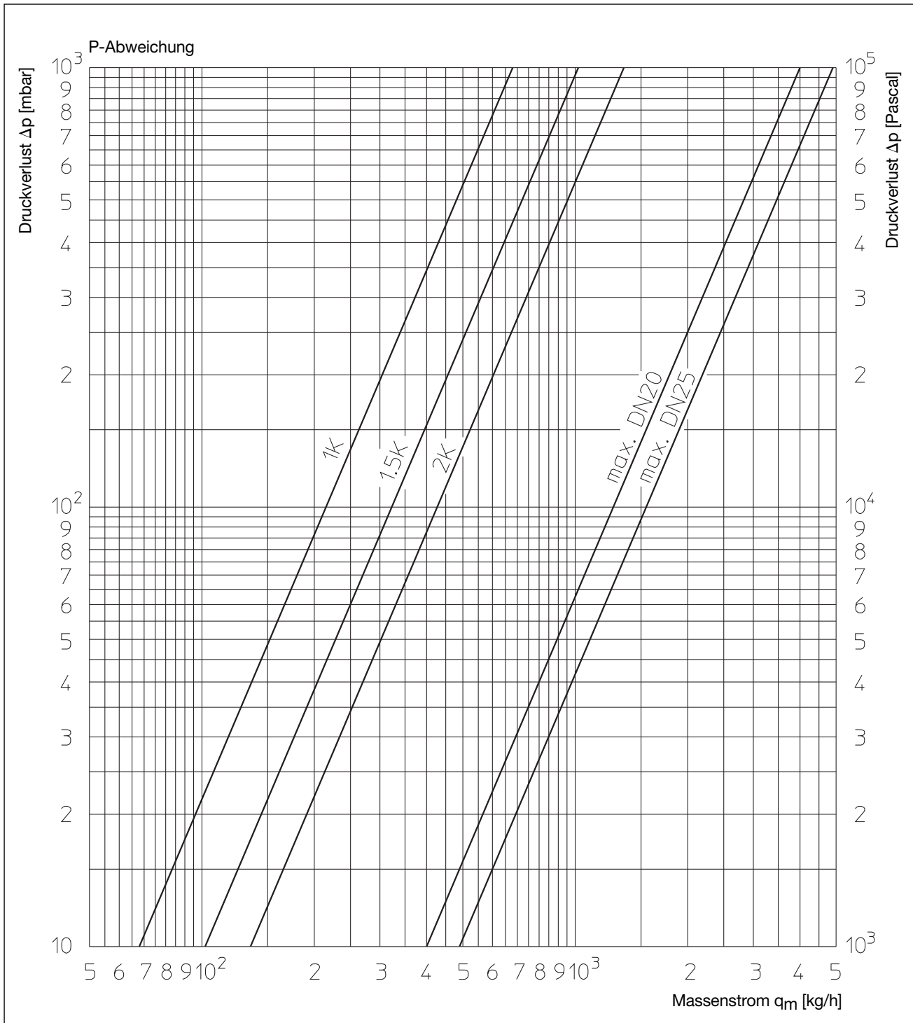
Diagramm 7 Oventrop Thermostatventile, „AZ H“
