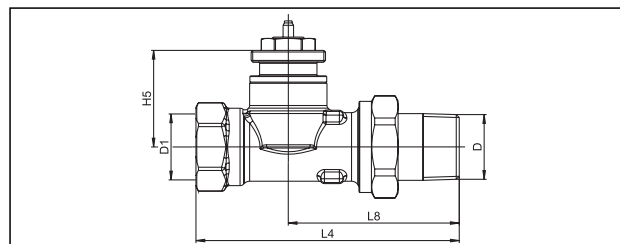
Maße Durchgangventil
