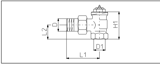
Maße Eckventil
