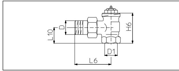
Maße Eckventil
