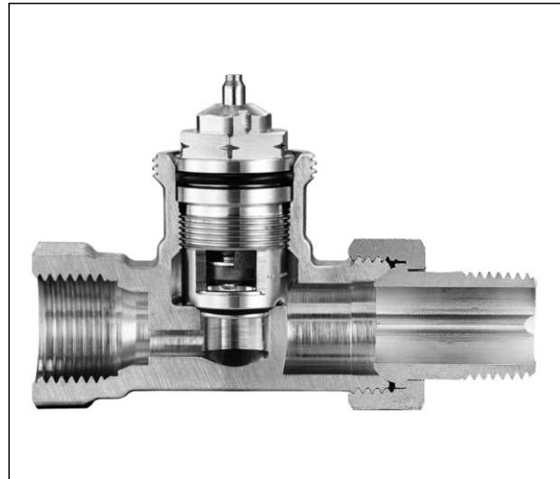
Durchgangsventil „AV 9“
